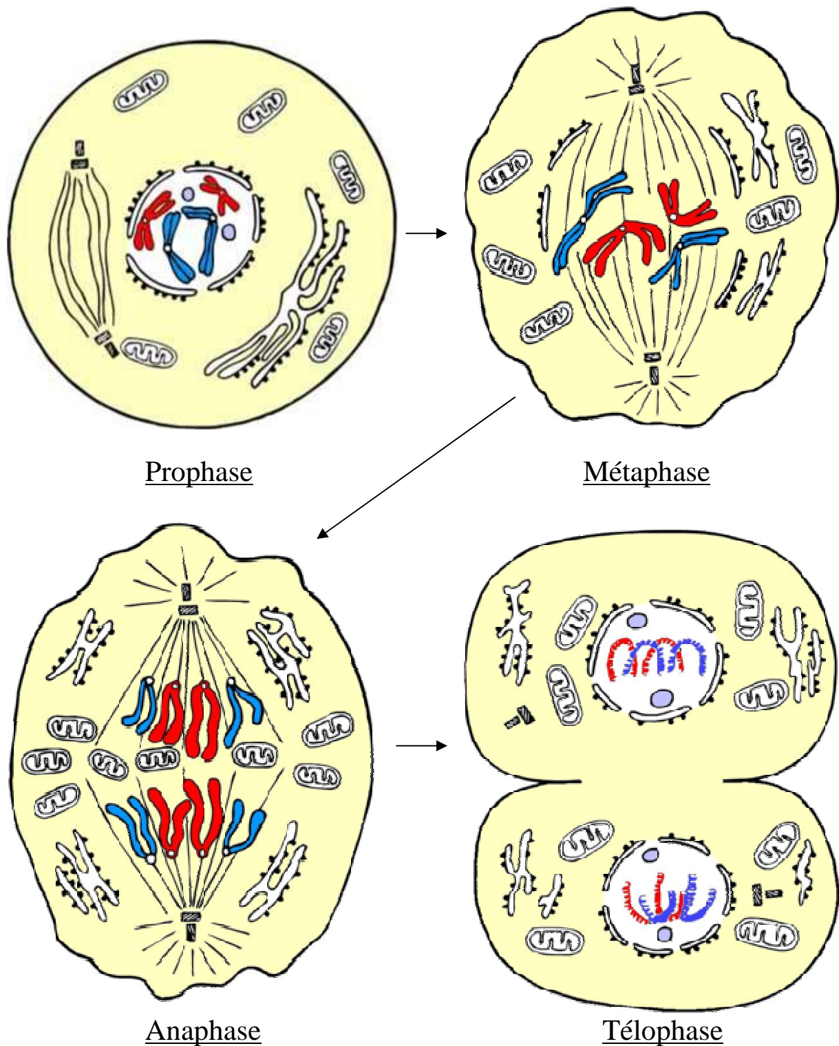
SCHÉMA 19 : MITOSE
