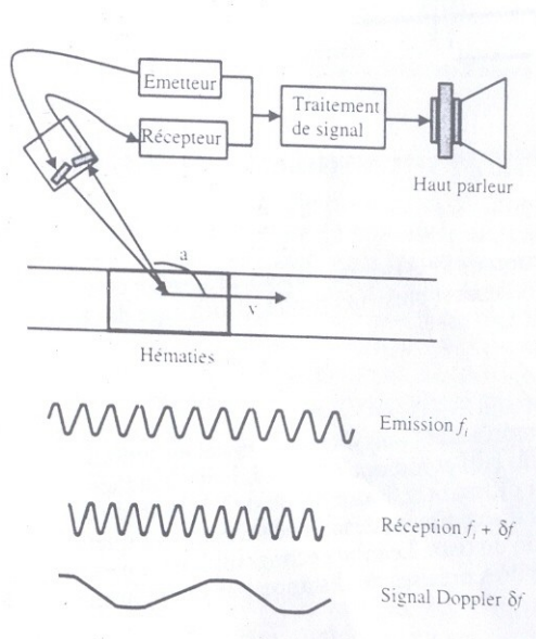
Fig. 3 : PRINCIPE DE L'EFFET DOPPLER
