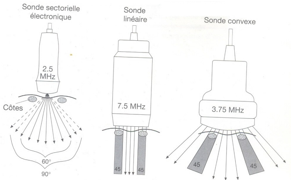
Fig. 6 Sondes électroniques
