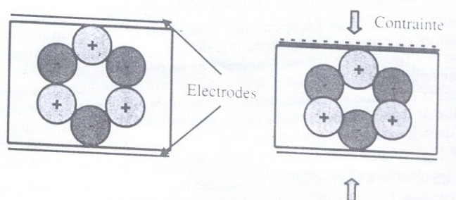
Fig. 4 : EFFET PIEZOELECTRIQUE.
