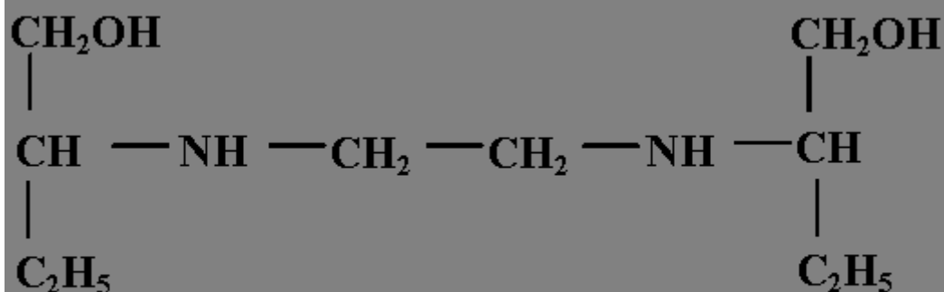
Fig.3:Structure de l'éthambutol
