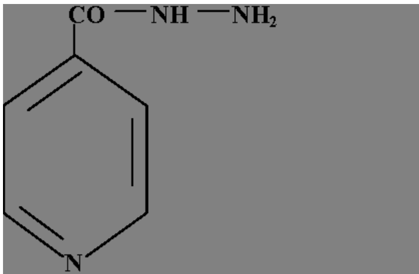
Fig. 2 Structure de l'Isoniazide [5]
